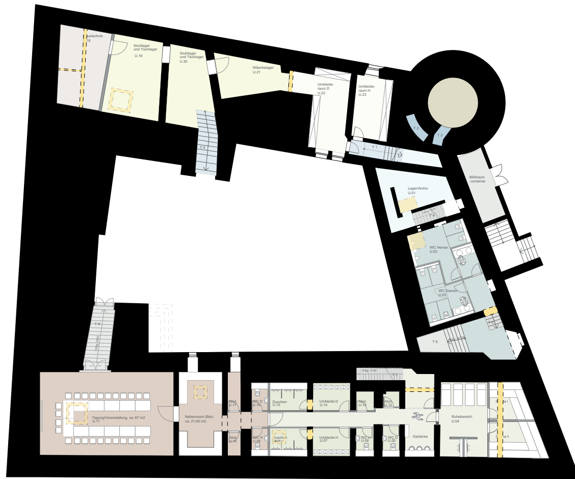
Untergeschoss
