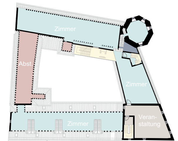
Funktionen 2.Obergeschoss
