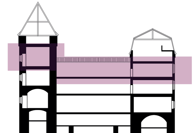
Schnitt
