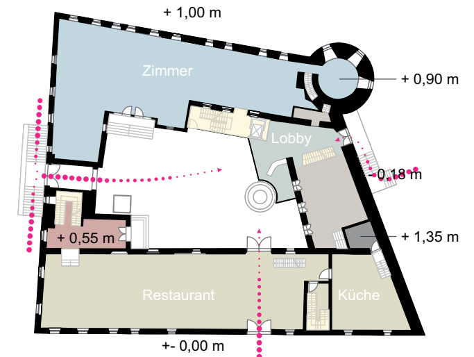
Funktionen Erdgeschoss
