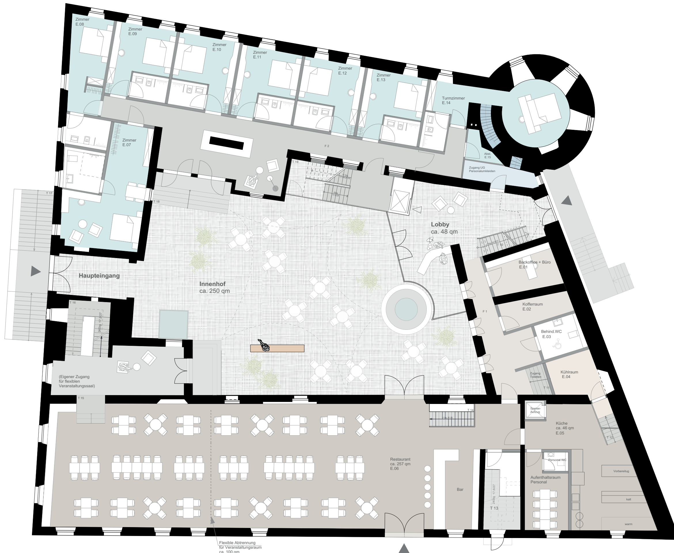
Funktionen Erdgeschoss
