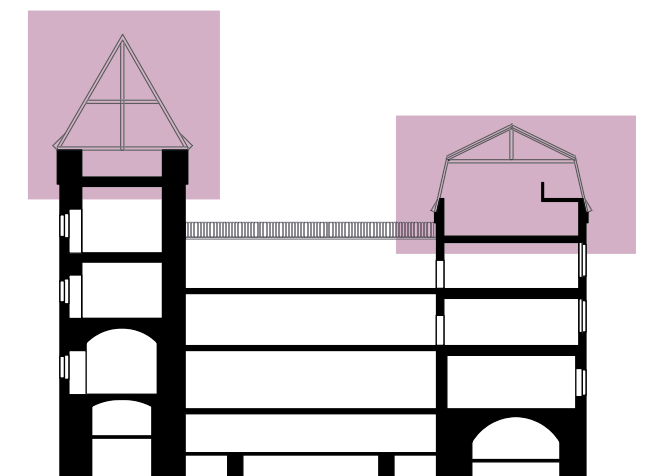
Schnitt
