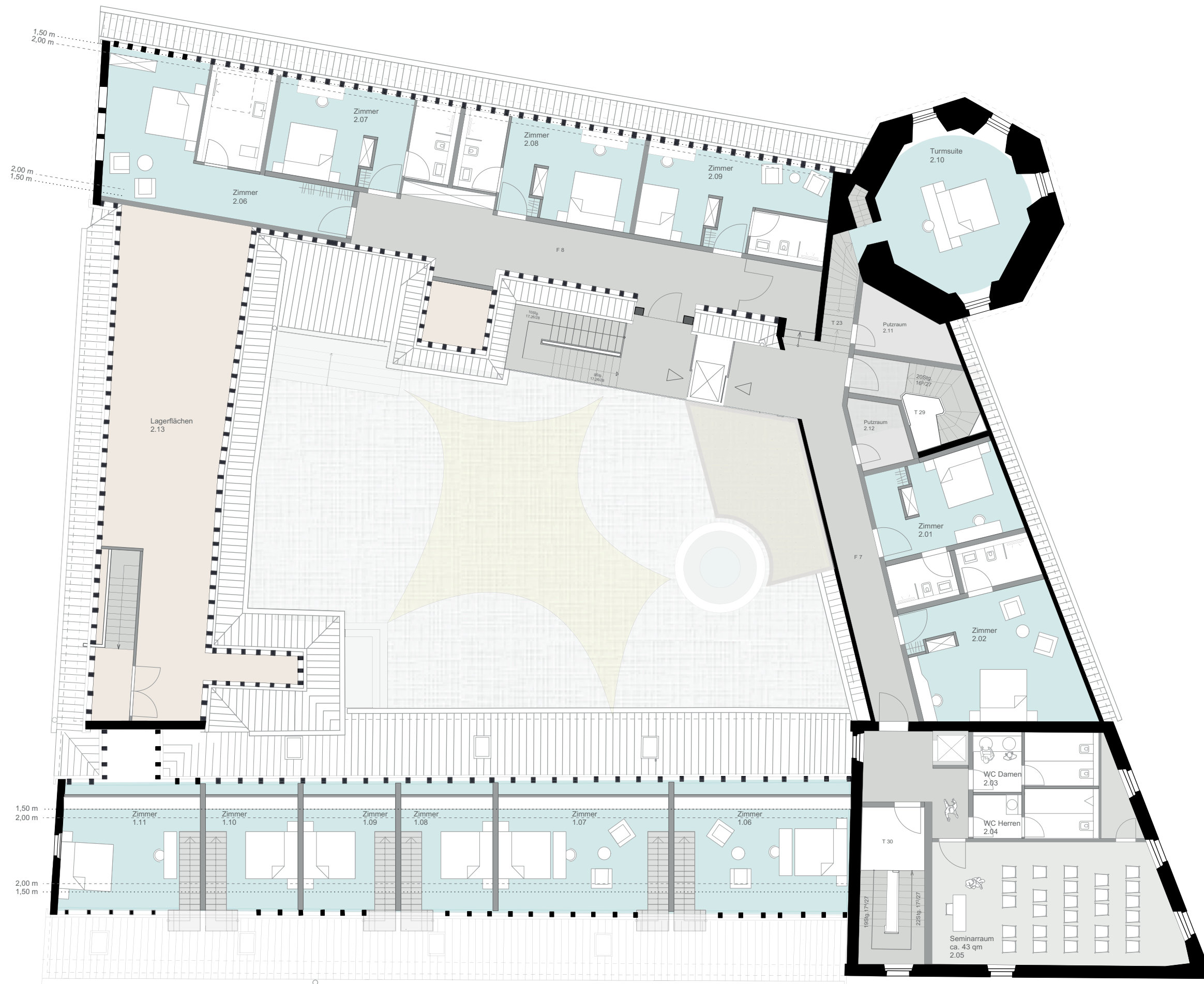
Funktionen 2.Obergeschoss
